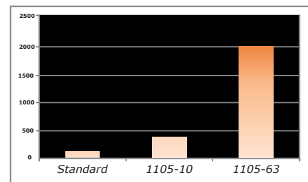
Otsonitesti (EN 27326), 40°C, 50 ppm
